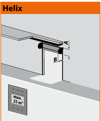
Helix spiraal A= 1100 mm B= 1200 mm Breedte max. 5000 mm Hoogte: min. 2500 mm max. 5000 mm
