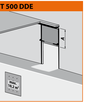
Système de rails vertical avec axe de ressort surbaissé A= hauteur du jour + 400 mm, B= non applicable Largeur est max. 3.200 mm Hauteur est max. 3.200 mm
