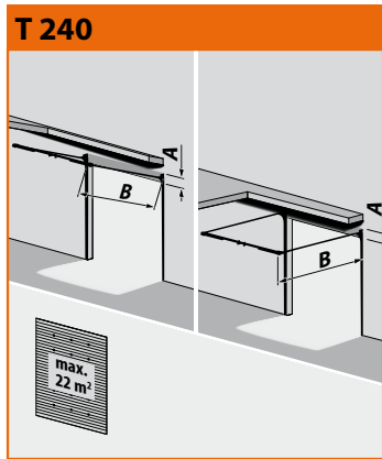
Système de rails à linteau réduit, câbles glissés à l'intérieur + profilé de support en acier A= 240 mm B= hauteur du jour + 1 000 mm Largeur est max. 6.500 mm
