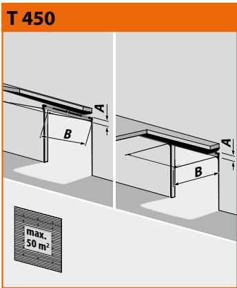
Système de rails normal (standard) A= 430 à 510 mm B= hauteur du jour + 650 mm
