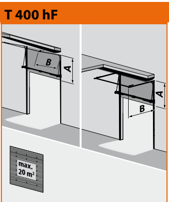
Système de rails levée semi-verticale avec axe de ressort surbaissé + profilé de support en acier A= élévation + 200 mm, B= hauteur du jour – élévation + 600 mm Largeur max. 4.500 mm Élévation min. 1.450 mm
